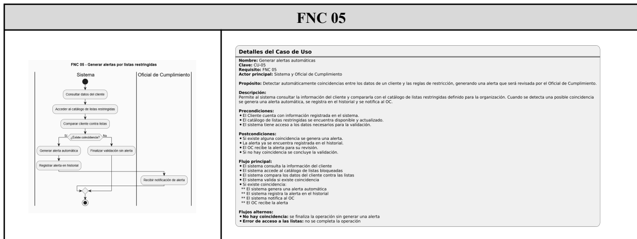
Figura 3. Detalles del Caso de Uso 05 y Diagrama de Actividades
