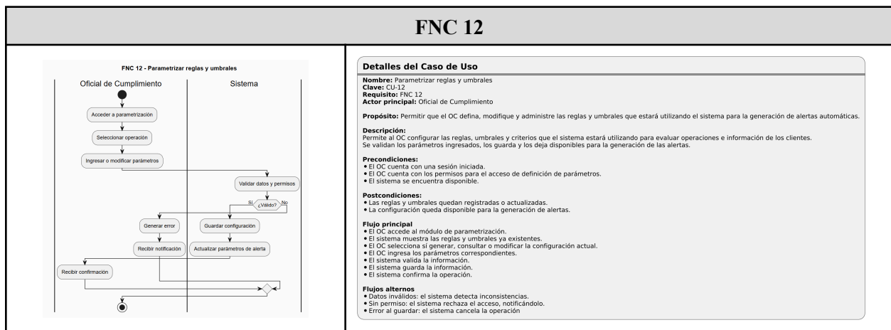
Figura 5. Detalles del Caso de Uso 12 y Diagrama de Actividades
